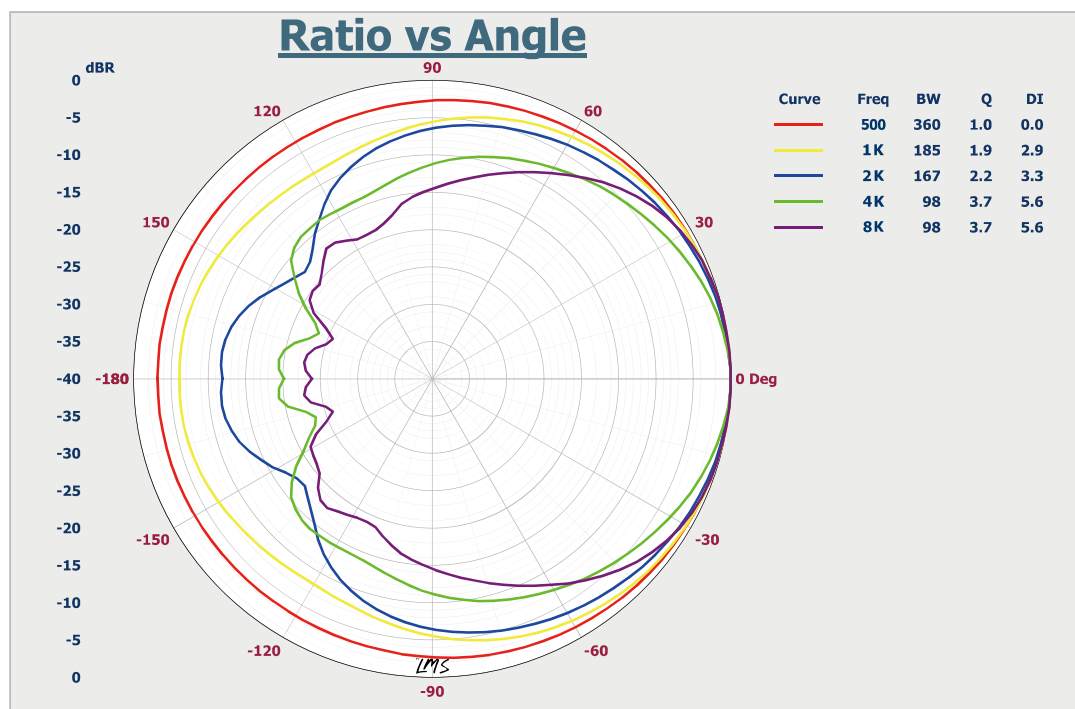
Круговая диграмма направленности громкоговорителя LPA-30K
